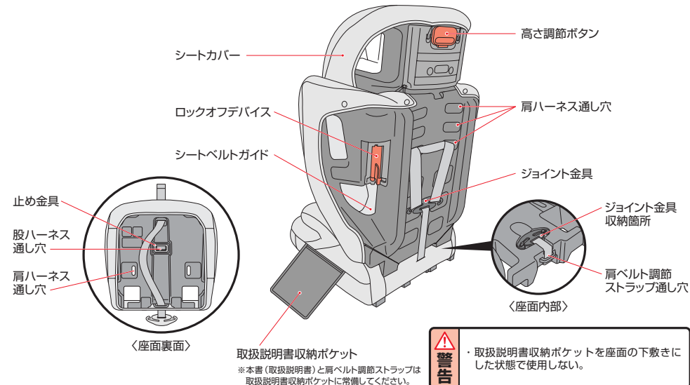
〈本体背面〉
